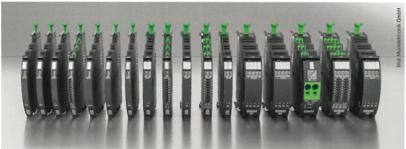
Bild 2 | Bei Micro Pro handelt es sich um ein modulares System zur Stromüberwachung und Potenzialverdrahtung.
